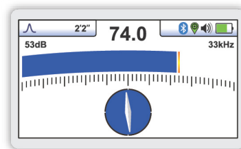
Écran classique - Affiche un signal max lors de la localisation. L'indicateur du compas devient bleu lorsqu'il est dans l'axe du réseau.
