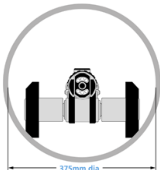
CPL 150 avec des grandes roues de 140mm (déplié)
